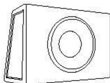
Geschlossen/Sealed 26.4 Liter Reflex/Vented 47.0 Liter 7 x 18 cm CP* (1x)
