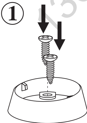
Abbildung 4 Aufbau Hochtöner Figure 4 Surface mount of Tweeter
