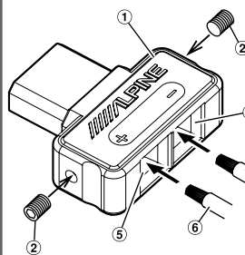
Lead end side of the product/ Côté extrémité du conducteur du produit/ Extremo del conductor del producto
