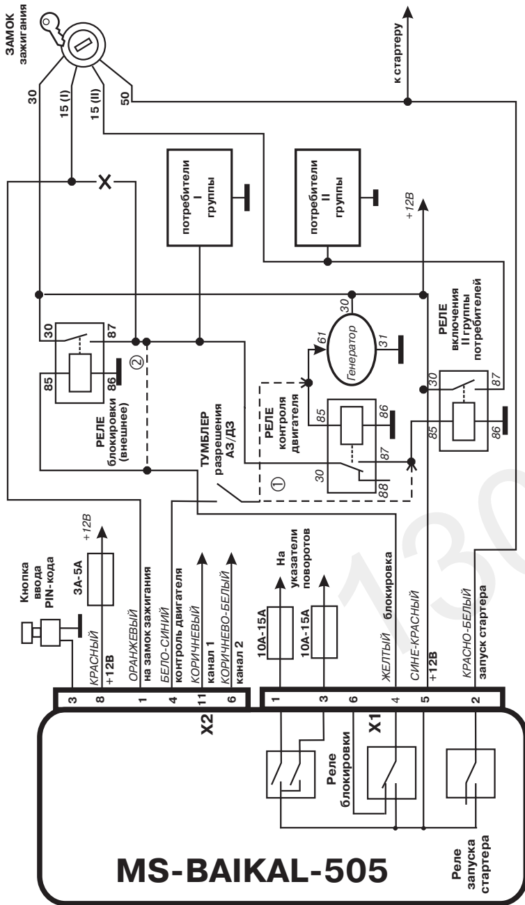
Рис.5. Реализация дистанционного и автоматического запуска (А3/Д3) ① Бело-синий провод входа контроля двигателя (X2.4) можно подключать непосредственно к клемме 61 ② Если ток в цепи блокировки зажигания (X1.4) превышает 5 А, то для включения потребителей 1-й группы должно использоваться внешнее реле.
