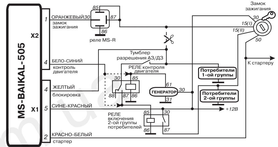
Если ток в цепи блокировки зажигания (X1.4) превышает 5 А, то для включения потребителей 1-й группы должно использоваться внешнее реле. Бело-синий провод входа контроля двигателя (X2.4) можно подключать непосредственно к клемме 61 генератора
