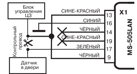
Рис. 10. Схема подключения к центральному замку, которому для отпирания требуется отрицательный импульс, а для запирания - разъединение проводов
