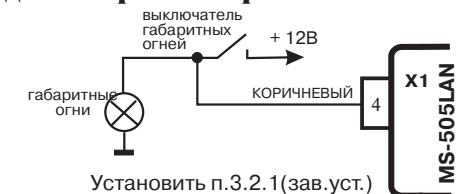
Рис. 17. Подключение сервисного входа для контроля габаритных огней
