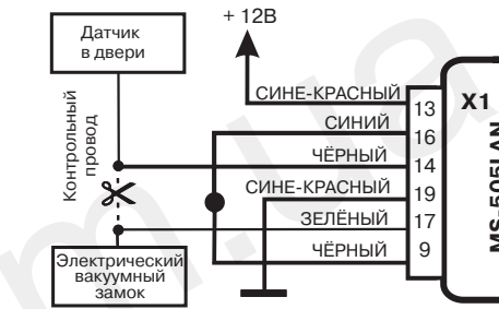
Рис. 9. Схема подключения к вакуумному центральному замку
