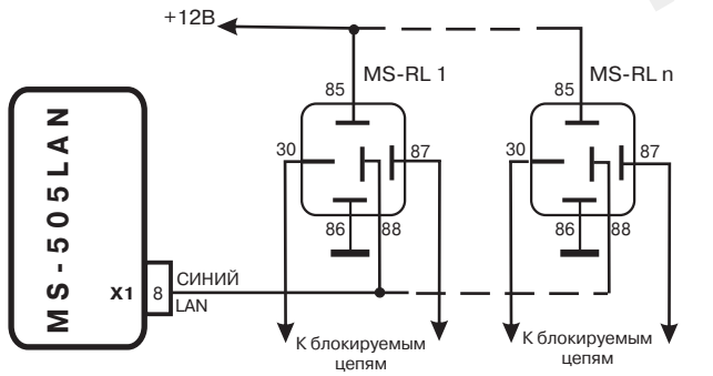
Рис. 15. Схема подключения реле блокировки MS-RL
