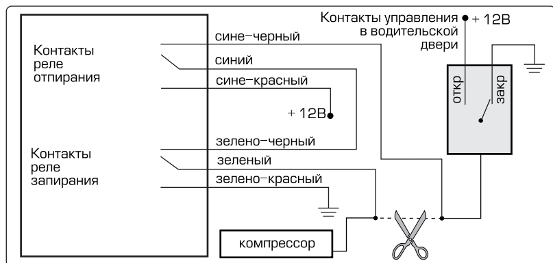
Схема подключения к пневматической системе запираения
